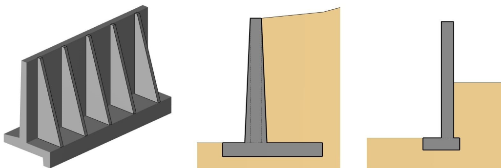
esempi di muri a mensola
