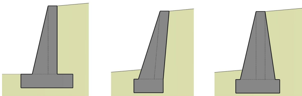
esempi di muri a gravità
