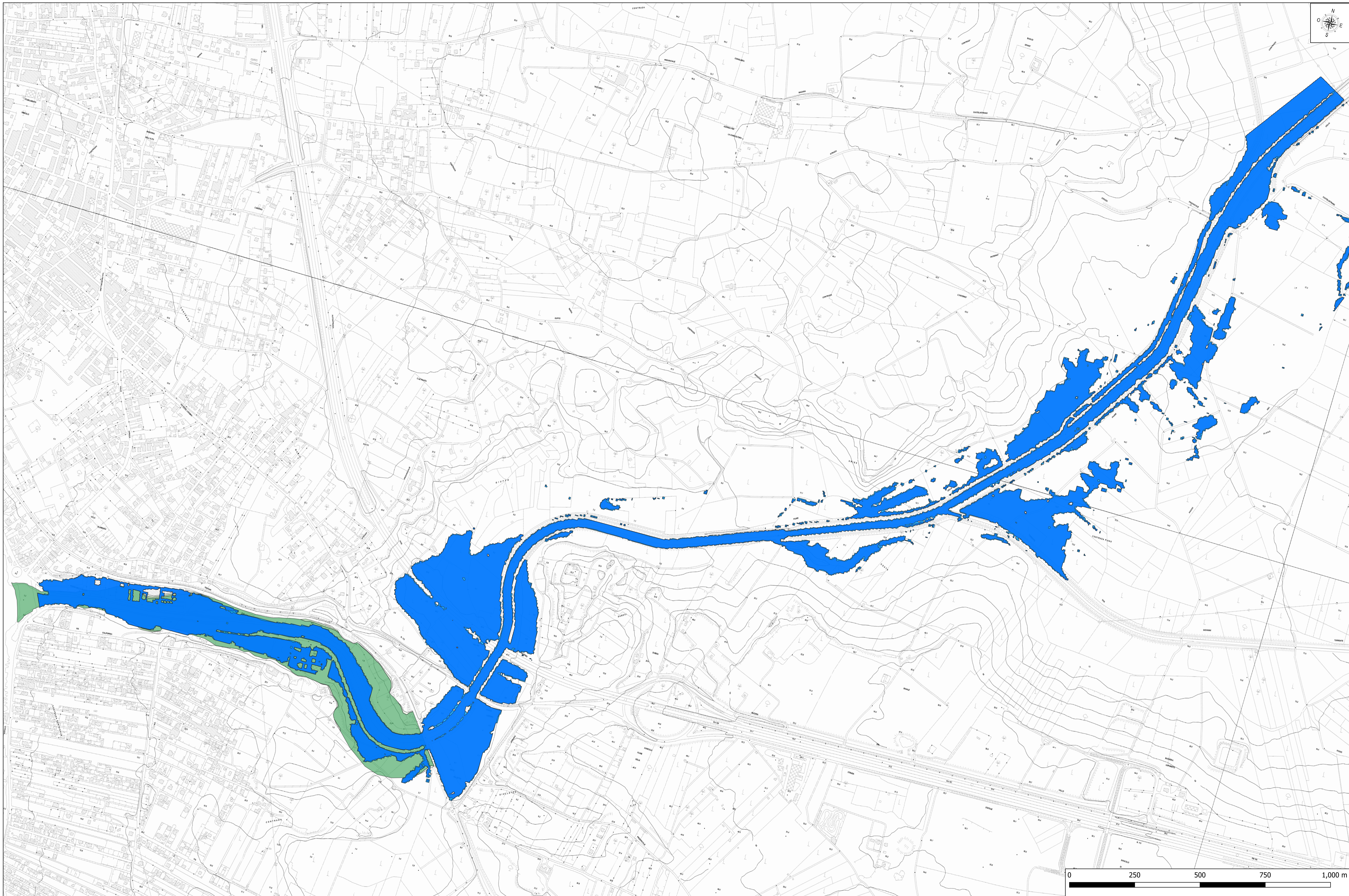
FIUME ARENA - AREE SUSCETTIBILI DI ALLAGAMENTO - Tr = 300 anni CARTOGRAFIA: Carta Tecnica Regionale Fonte: https://map.sitr.regione.sicilia.it/gis/services/ctr_10000/ctr_2013_base/MapServer/WMS/Server
