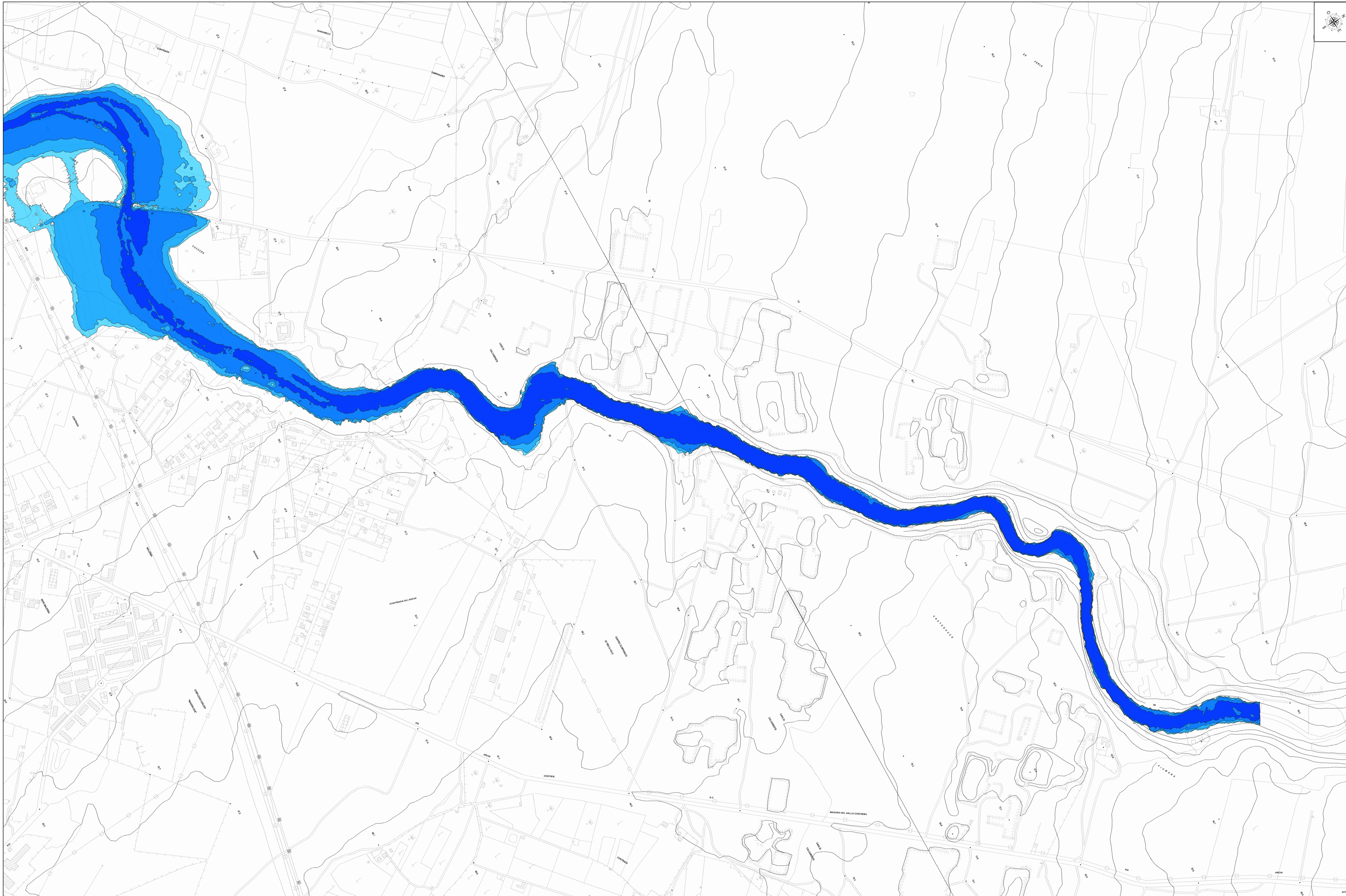
FIUME MAZARO - AREE SUSCETTIBILI DI ALLAGAMENTO - Tr = 300 anni - Scala 1:5000 CARTOGRAFIA: Carta Tecnica Regionale Fonte: https://map.sitr.regione.sicilia.it/gis/services/ctr_10000/ctr_2013_base/MapServer/WMS/Server
