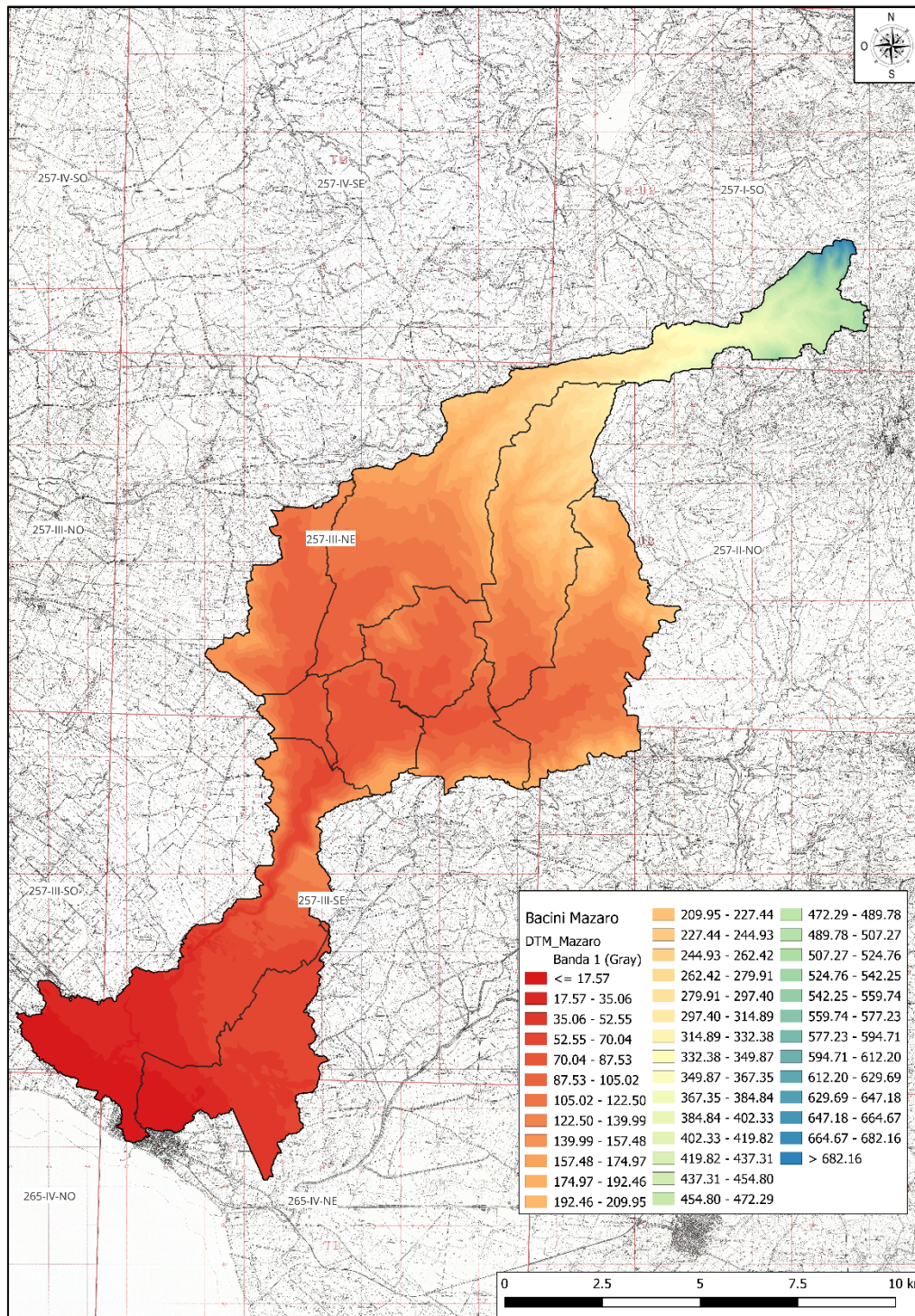
Fig. 10. Modello Digitale del Terreno - Bacino Fiume Mazaro
