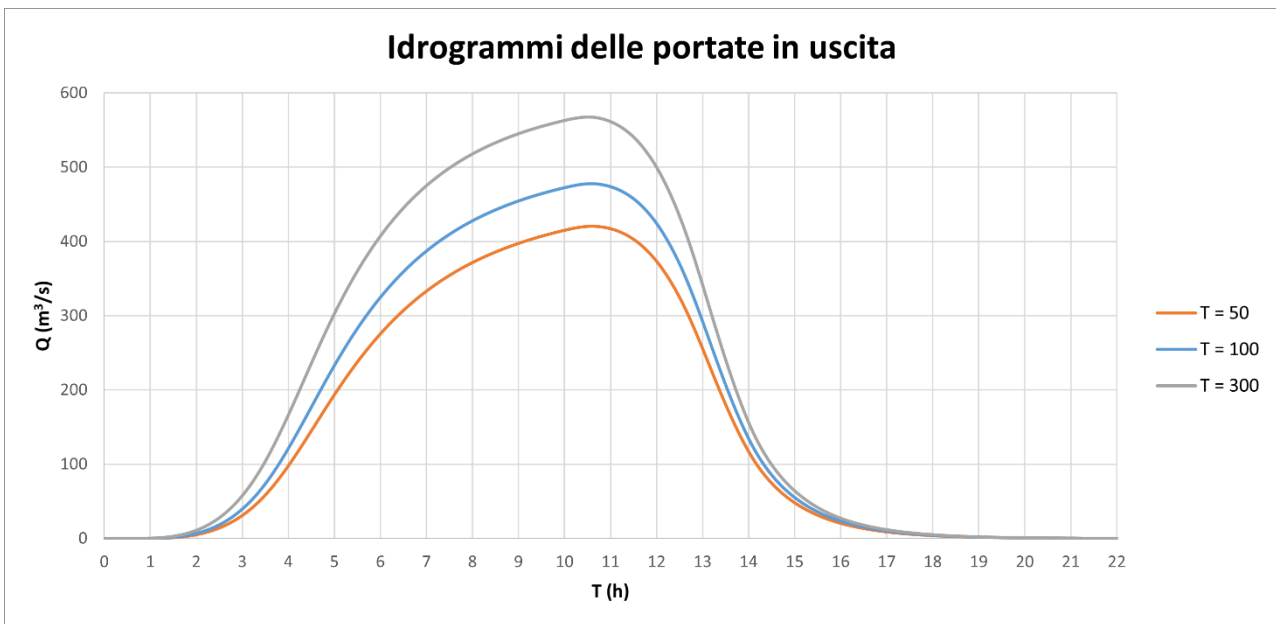
Fig. 18. Idrogrammi delle portate in uscita alla foce del Fiume Arena
