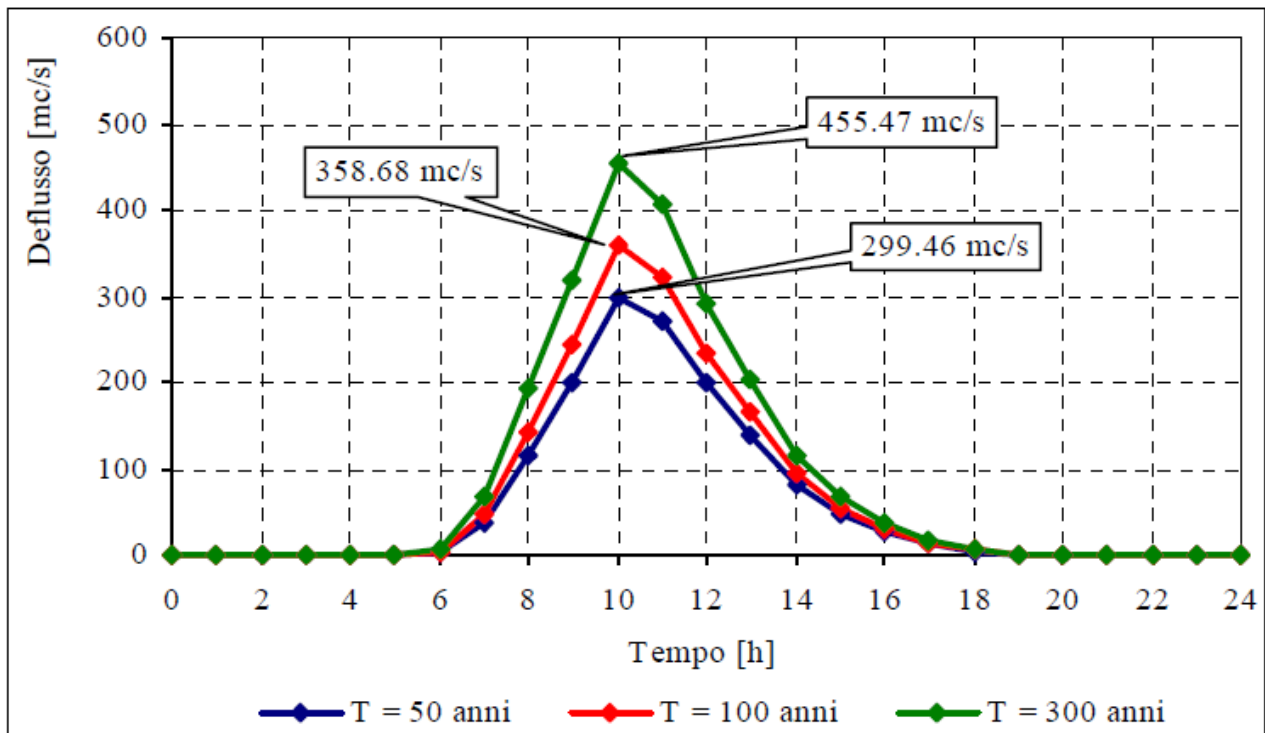
Fig. 14. Idrogrammi delle portate in uscita alla foce del Fiume Mazara (fonte: P.A.I.)
