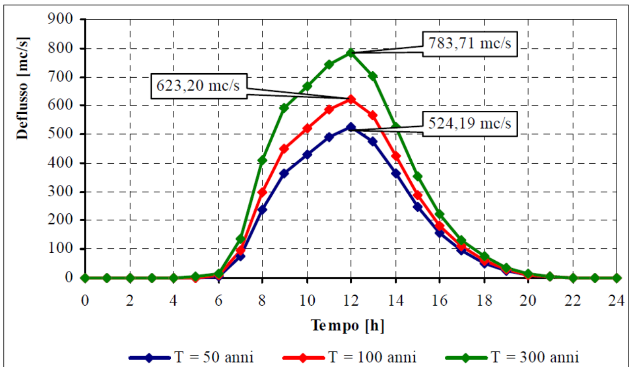
Fig. 19. Idrogrammi delle portate in uscita alla foce del Fiume Arena (fonte: P.A.I.)
