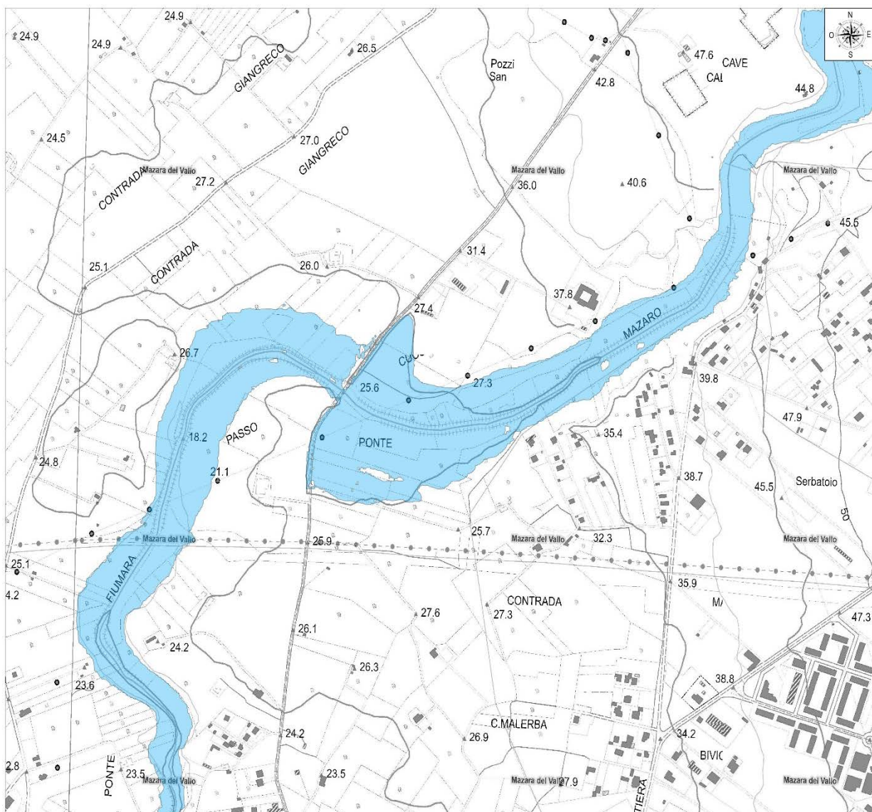
Fig. 23. Aree Suscettibili di Allagamento – F. Mazaro – Tr = 50 anni
