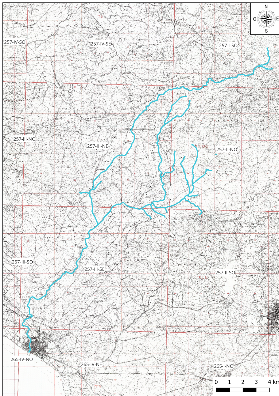
Fig. 4. Reticolo idrografico - Area fiume Mazaro
