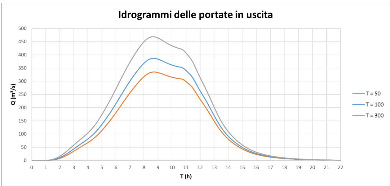
Fig. 13. Idrogrammi delle portate in uscita alla foce del Fiume Mazaro
