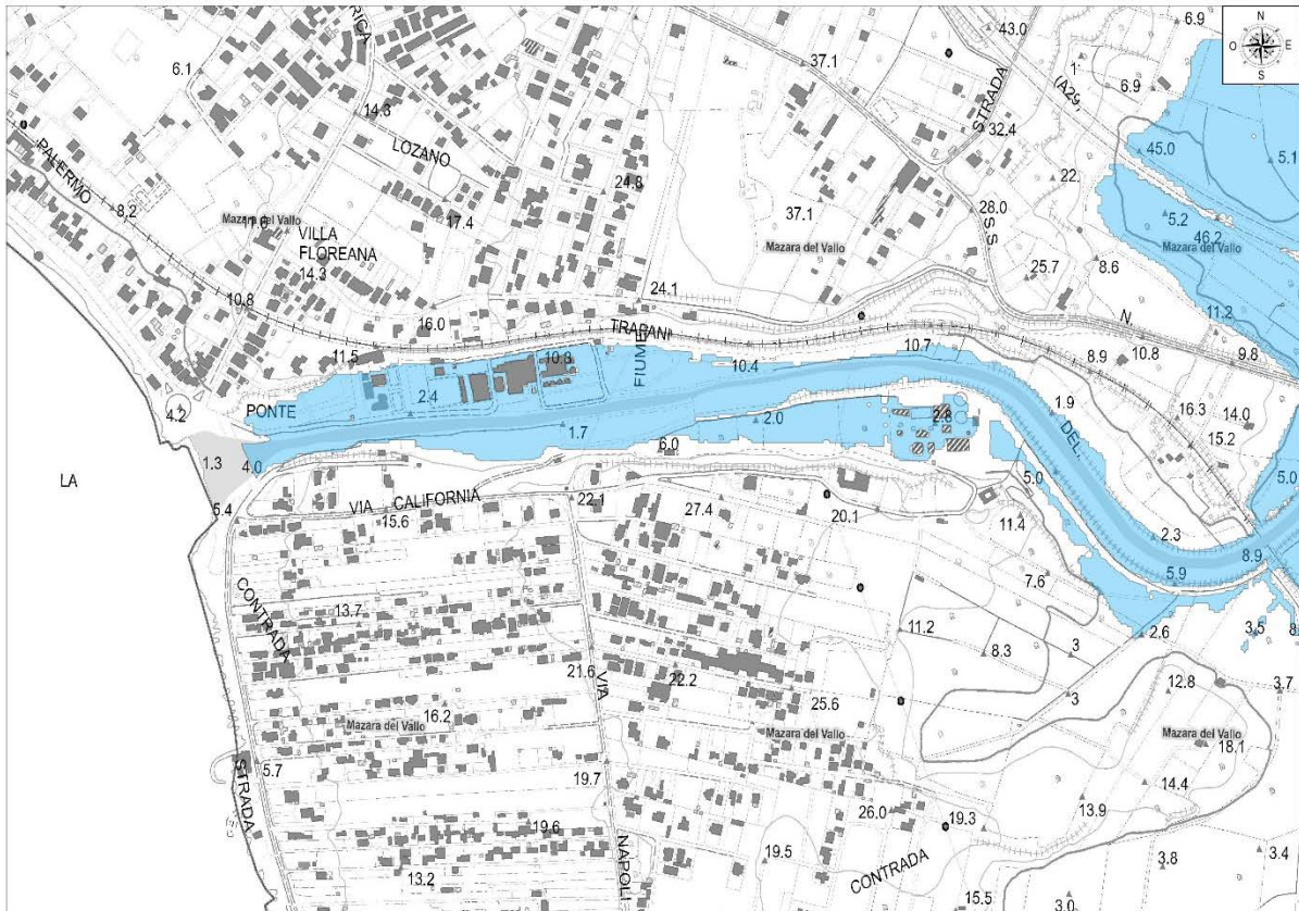
Fig. 29. Aree Suscettibili di Allagamento - Zona Est - Tr = 50 anni
