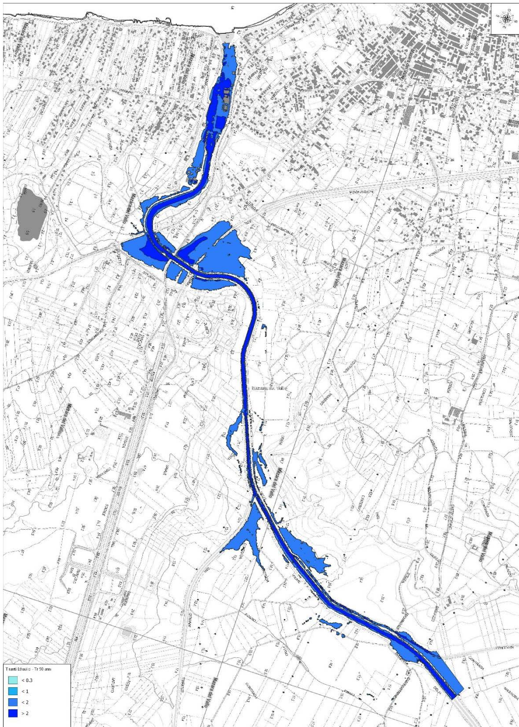
Fig. 22. Modellazione Idraulica Fiume Arena - Tr = 50 anni
