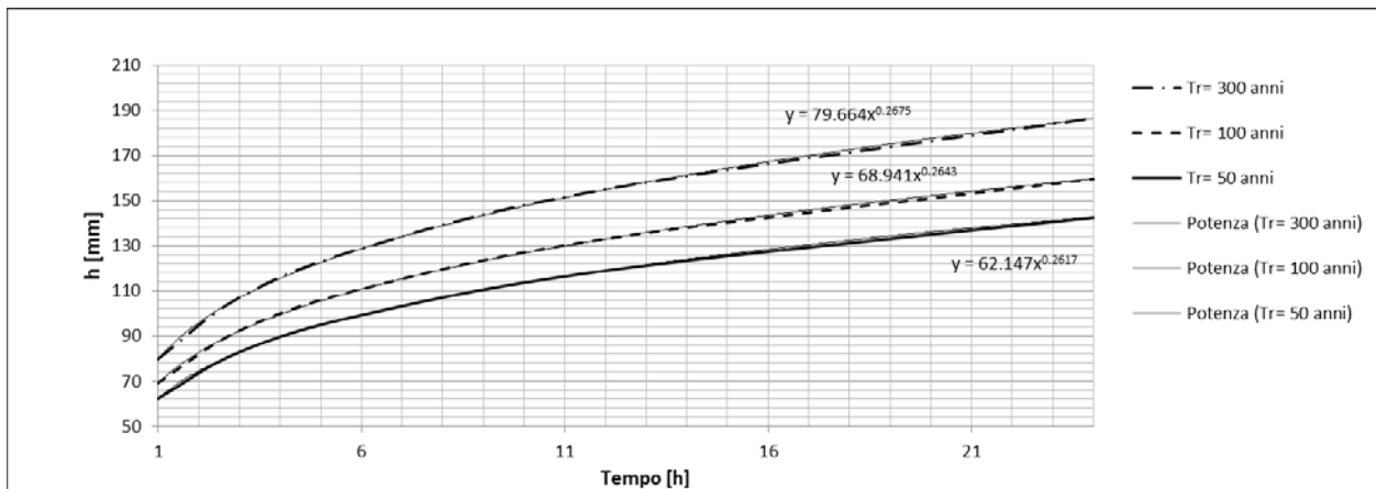
Fig. 17. Curva di probabilità pluviometrica bacino Fiume Arena
