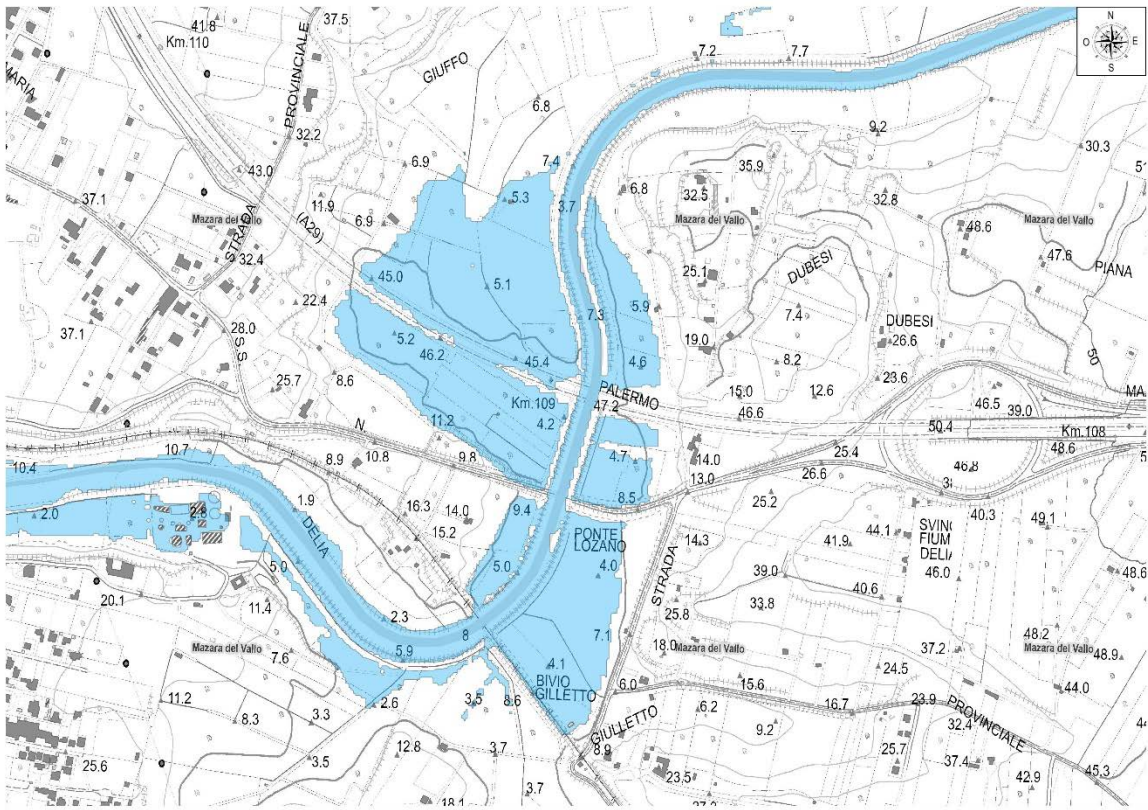
Fig. 27. Aree Suscettibili di Allagamento – attraversamenti E90 e SS115 - Tr = 50 anni
